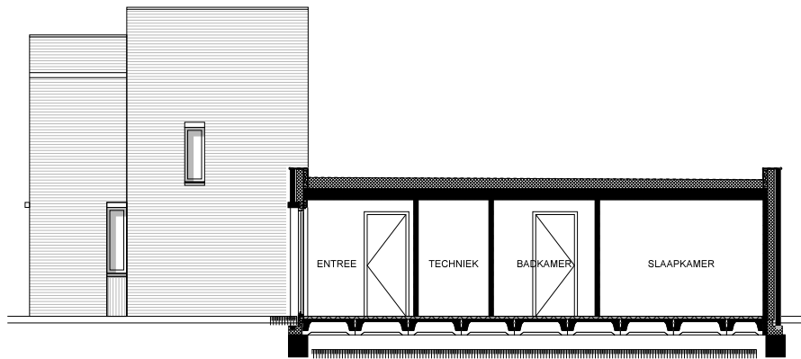
ACHTERGEVEL
