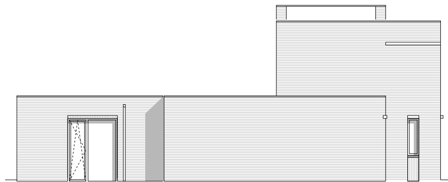
ZIJGEVEL / DOORSNEDE B-B
